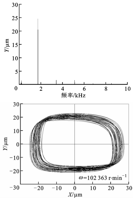
图 7 最高转速下转子的振动信号
