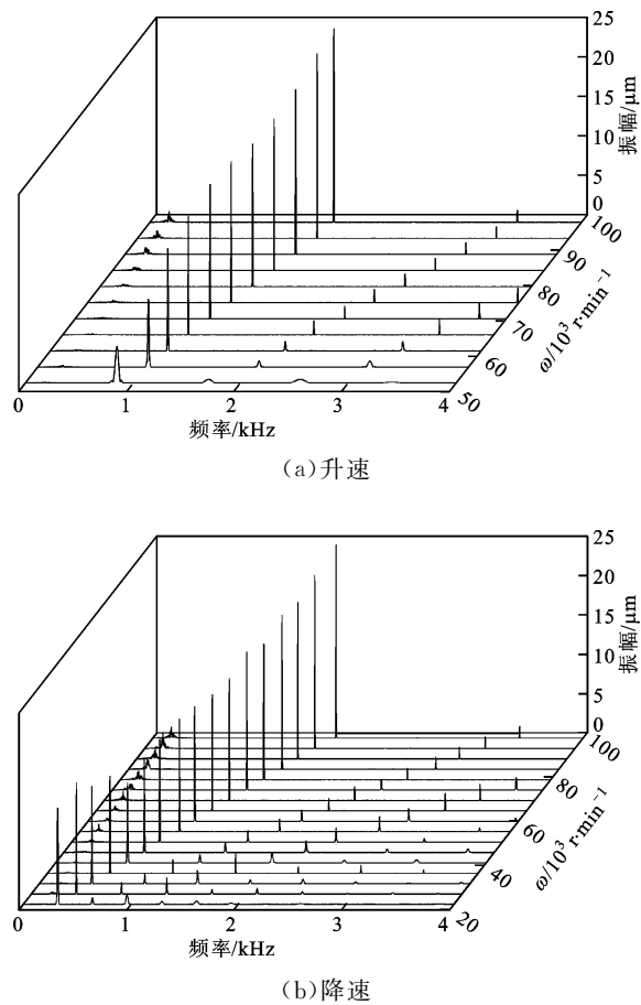
图 6 周叉轴叉排列方式下降降速瀑布图
