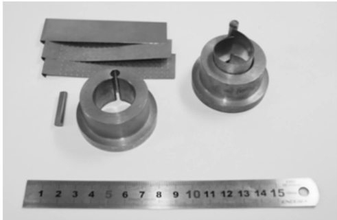
图 4 实验用箔片径向轴承
