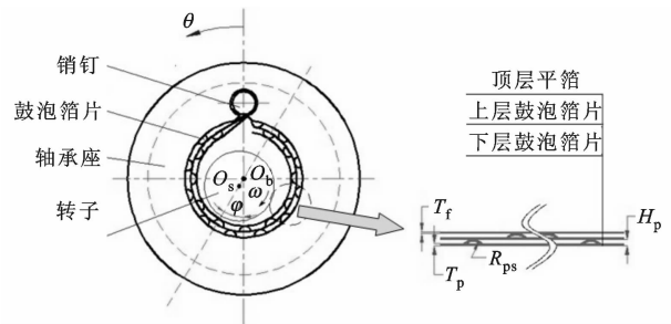
图 1 多层弹性支承箔片轴承原理图
