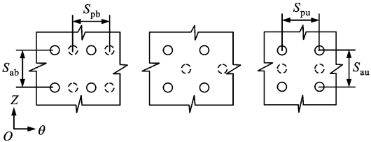
图 2 3 种典型的鼓泡位置结构
