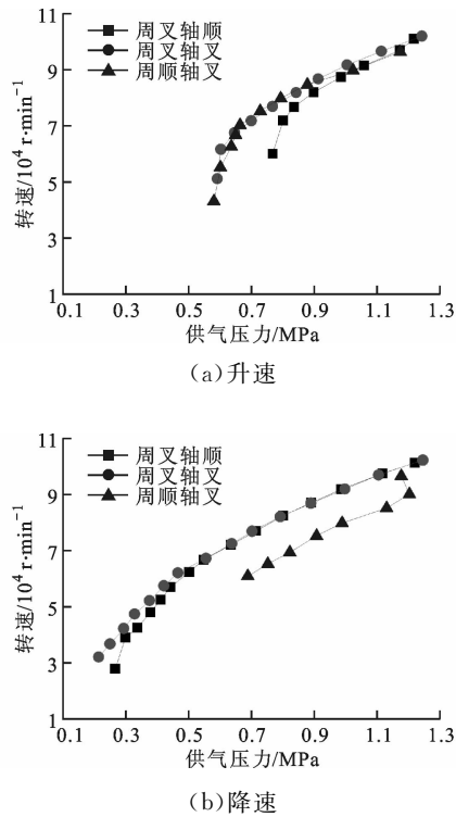
图 5 升降速过程中 3 种鼓泡相对位置下透平膨胀机转速与供气压力之间的关系
